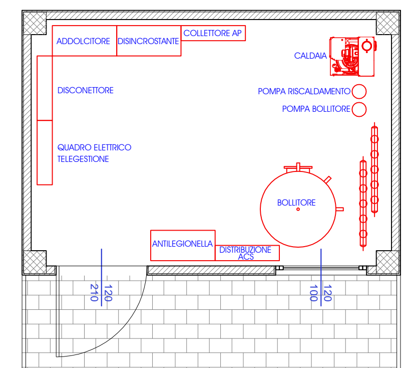
PIANTA CENTRALE TERMICA - SCALA 1:50 POSIZIONE INDICATIVA APPARECCHIATURE
