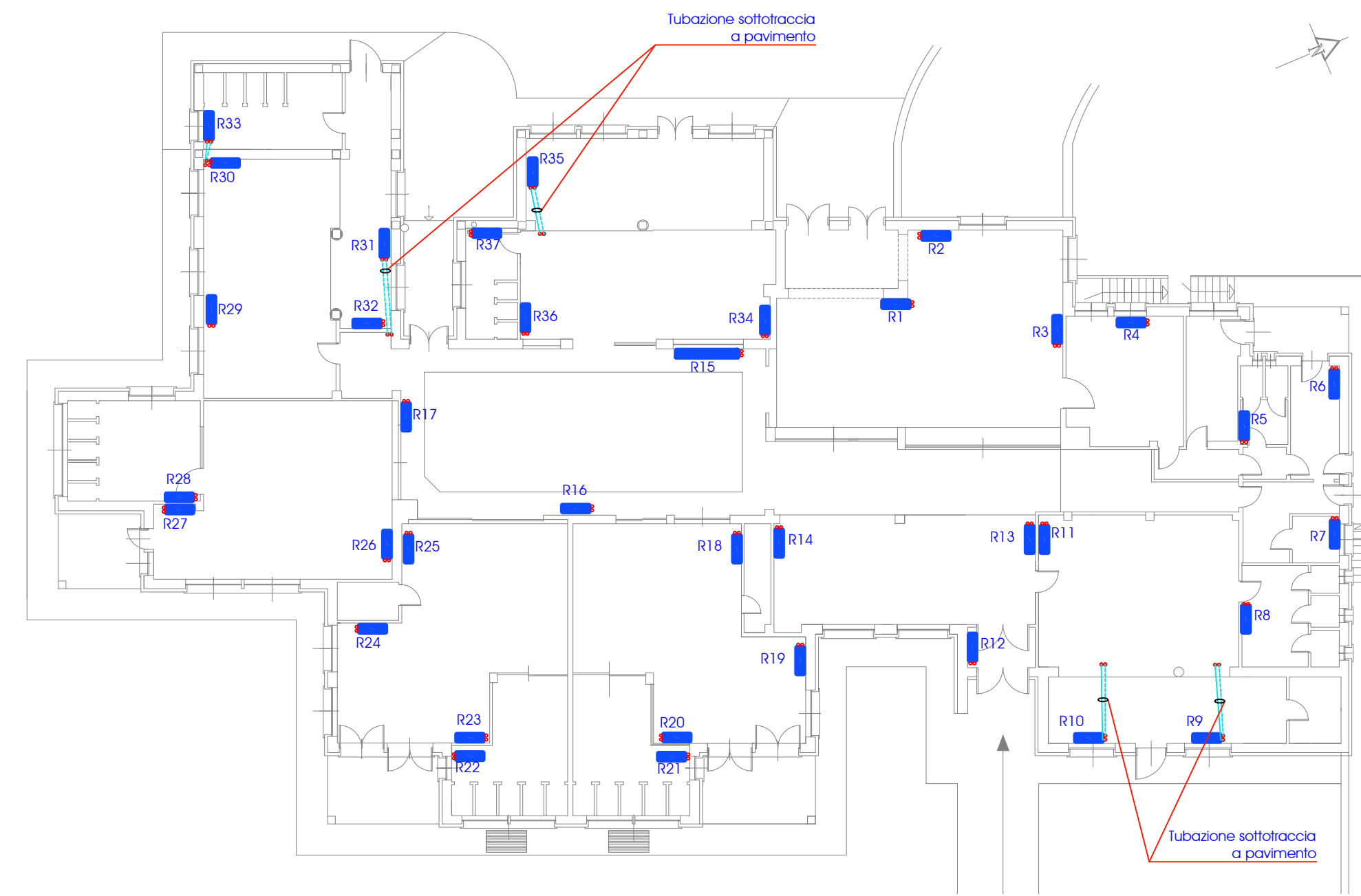
PIANTA PIANO TERRA - SCALA 1:200 DISTRIBUZIONE DEI TERMINALI DI RISCALDAMENTO E CONNESSIONI
