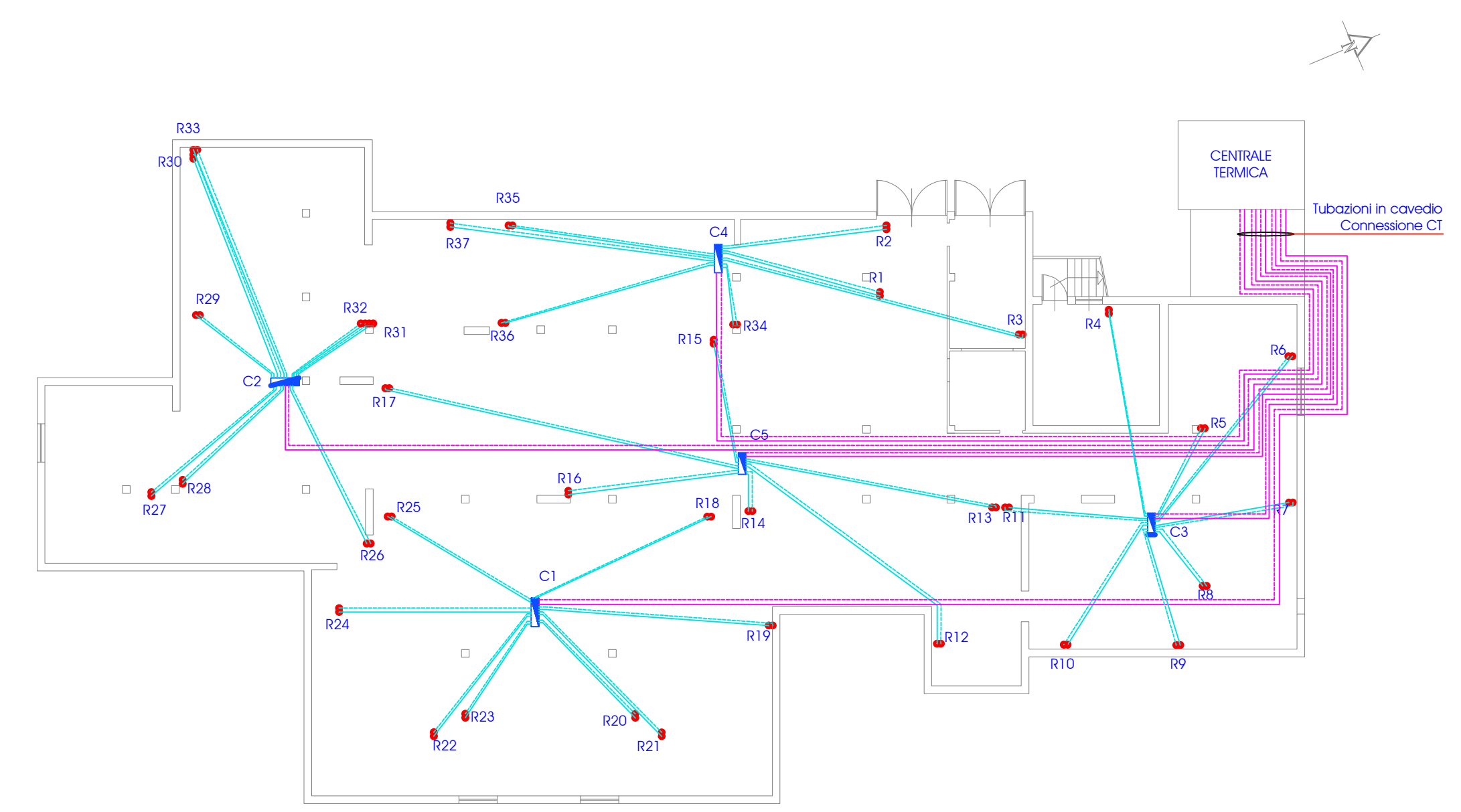
PIANTA PIANO INTERRATO - SCALA 1:200 DISTRIBUZIONE DELLE TUBAZIONI DELL'IMPIANTO DI RISCALDAMENTO e COLLETTORI DI DISTRIBUZIONE SINGOLE ZONE
